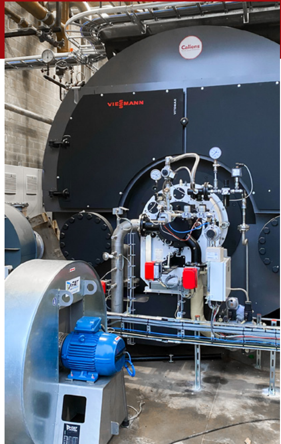
Hybride stoomketel van 9 T/h, verbranding geurgassen via brander
